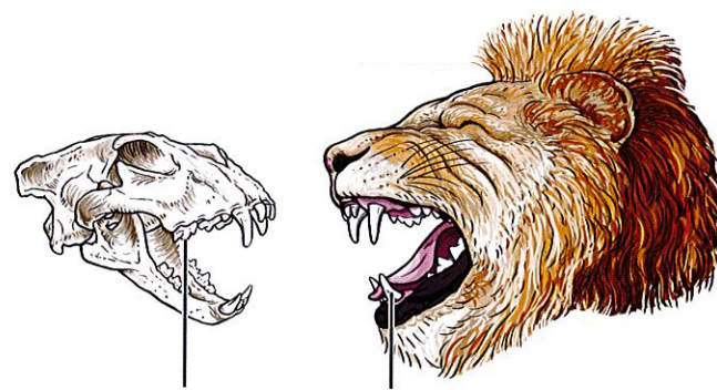
knipkies hoektand het gebit van vleeseters
